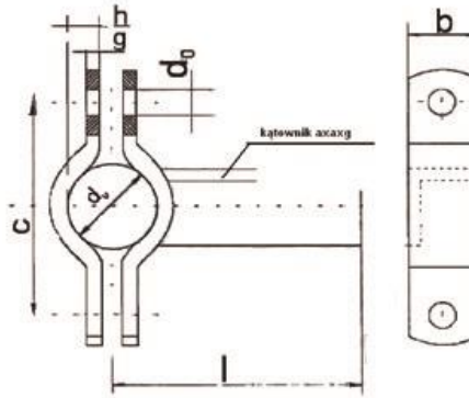
Uchwyt do rur typ „D” (Rohrhalter)
